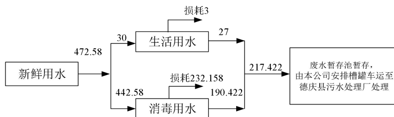
图 3-1 项目运营期水平衡图单位：t/a
